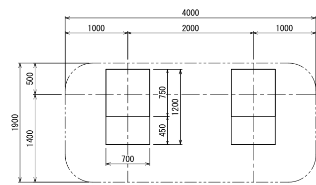
基礎伏図
