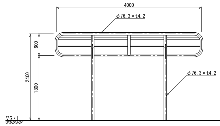
立面図
