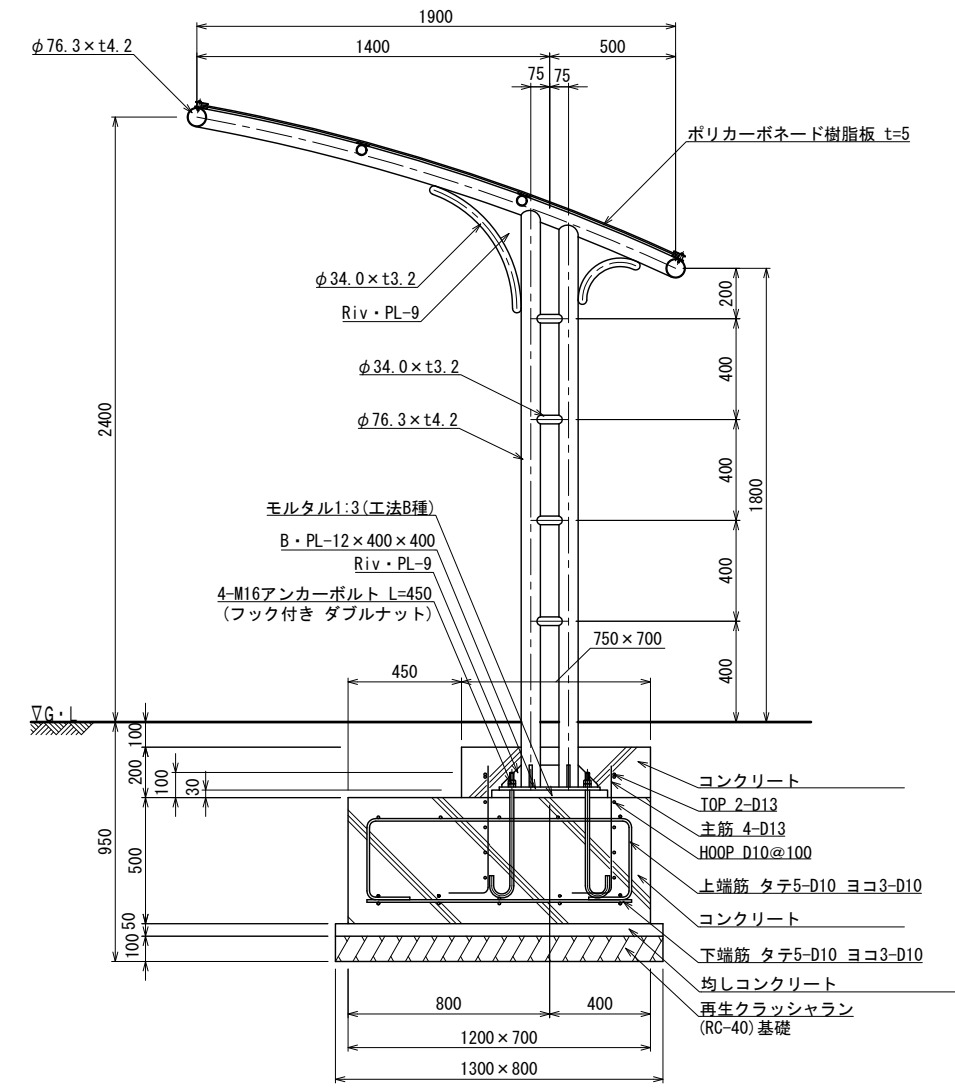
断面詳細図 S=1:15(A3 S=1:30)
