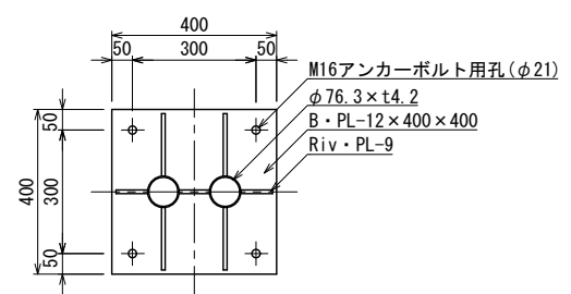
ベースプレート詳細図 S=1:10(A3 S=1:20)
