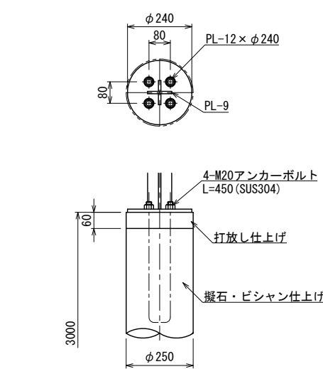
支柱上部取付詳細図 S=1:10 (A3 S=1:20)
