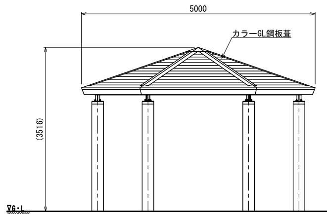
側面図
