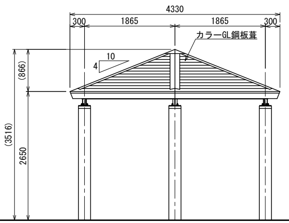
立面図
