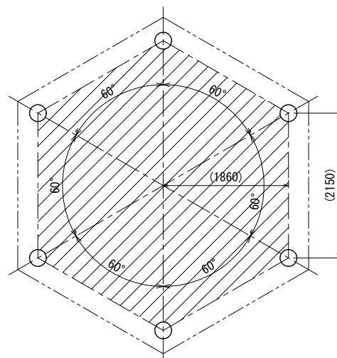
求積図
