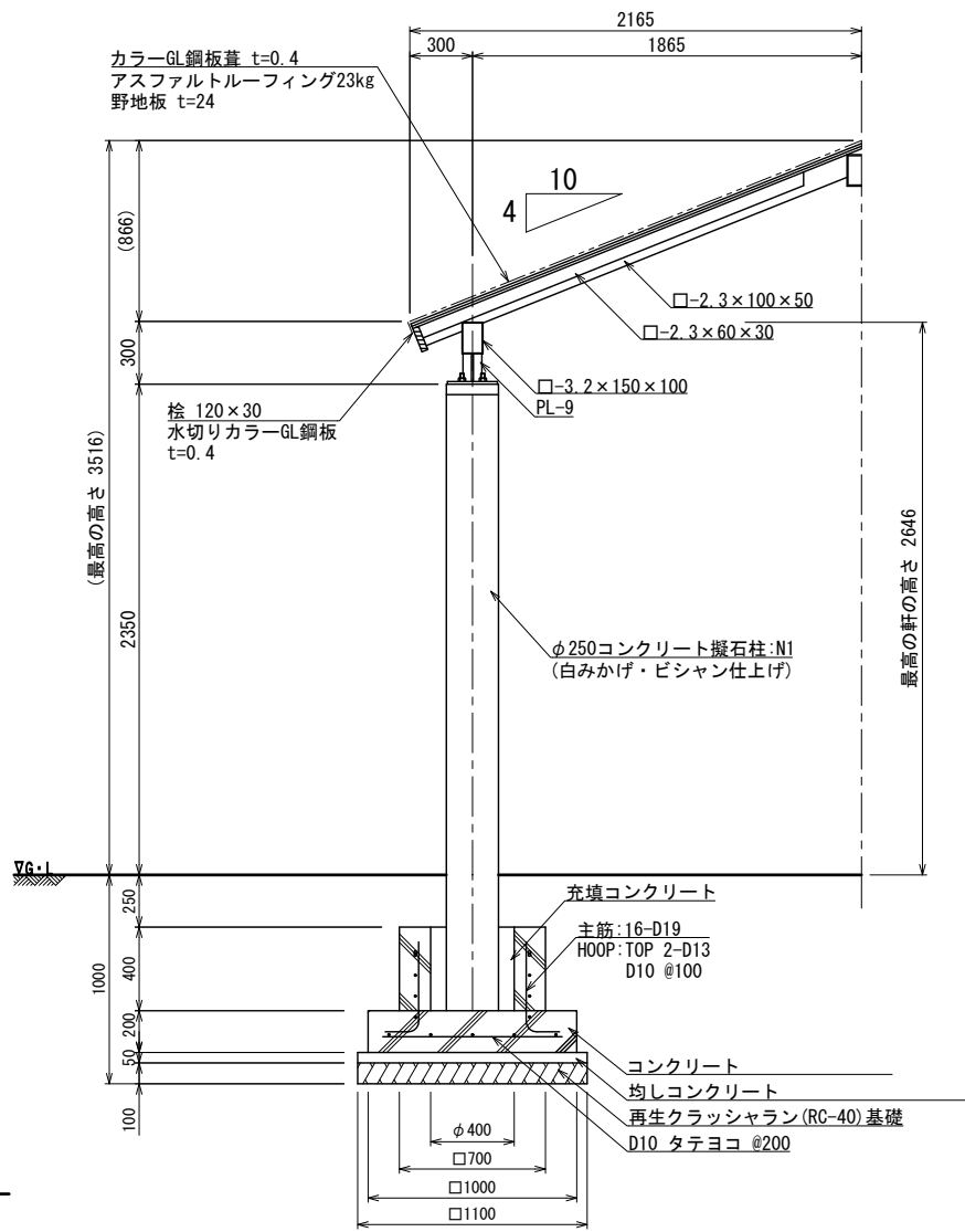
断面詳細図 S=1:20 (A3 S=1:40)
