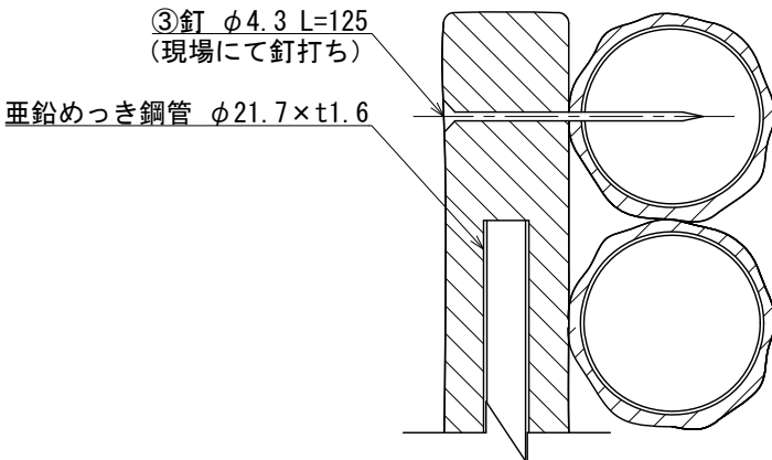
A-A' 断面図 S=1:4
