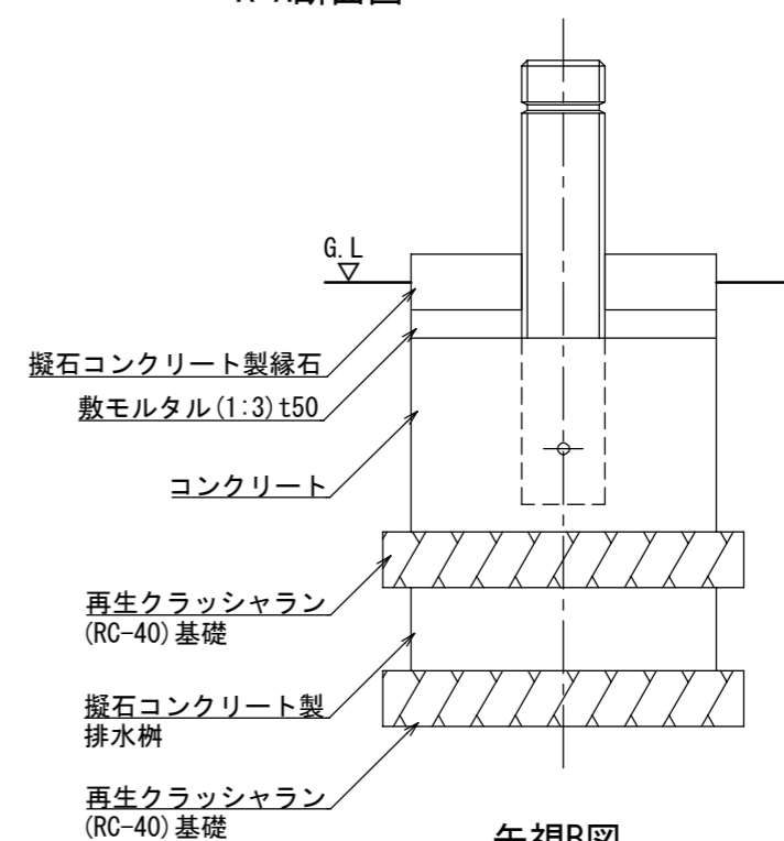
矢視B図
