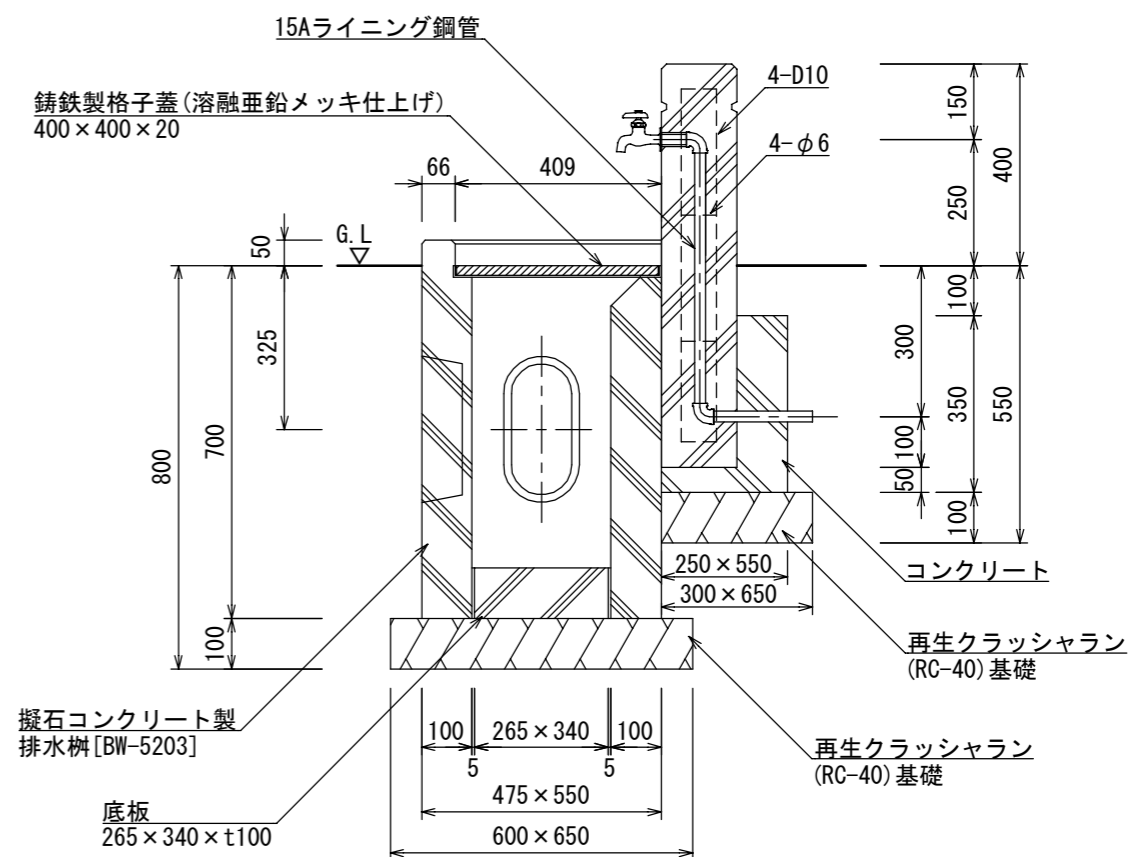
A-A断面図
