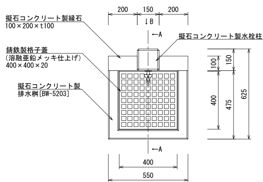
平面図
