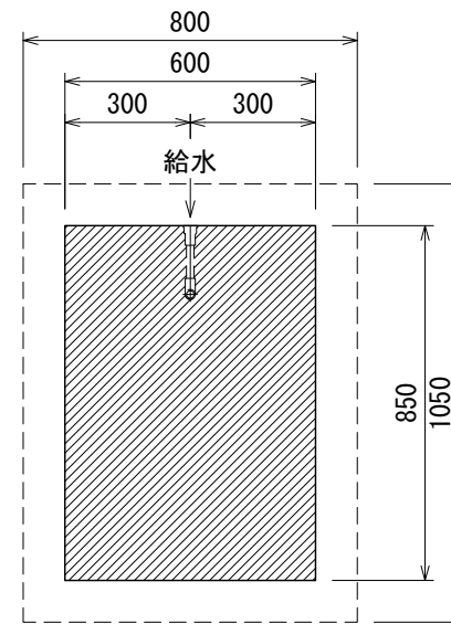
基礎伏図
