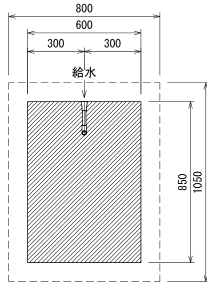
基礎伏図
