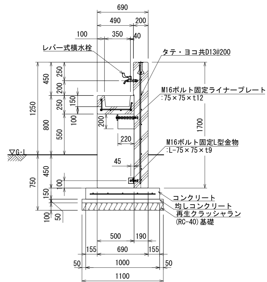
手洗い場 断面図
