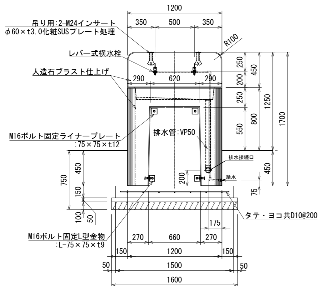
正面図
