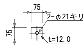
ライナープレート 詳細図 S=1:10
