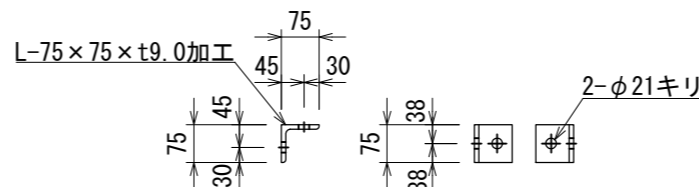
L型金物 詳細図 S=1:10
