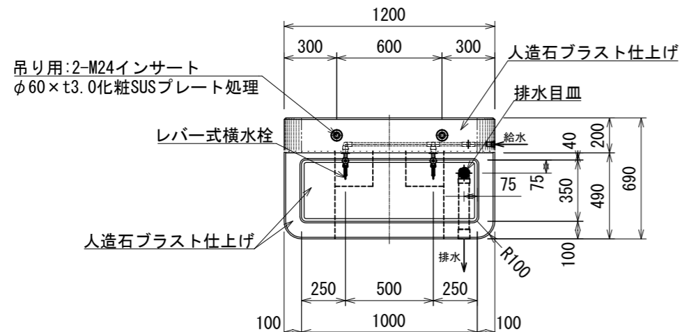
平面図
