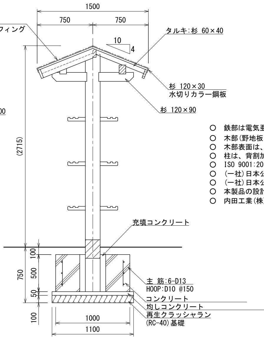
側面図
