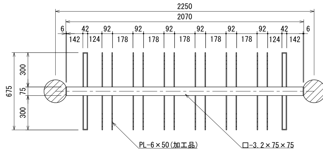
桶掛け金具詳細図 S=1:20
