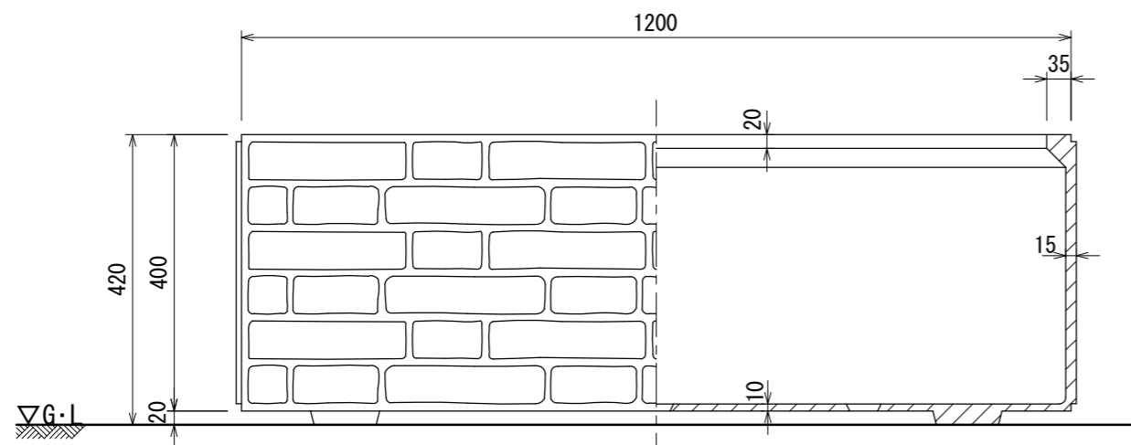
立・断面図
