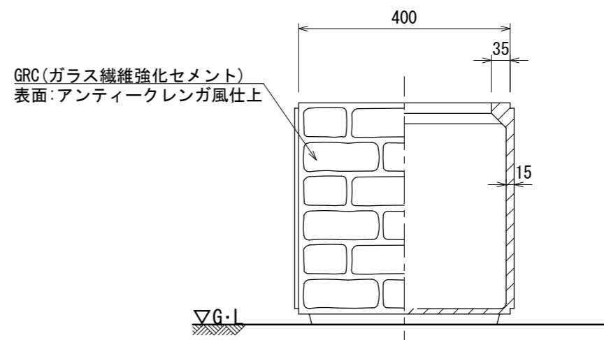
側・断面図
