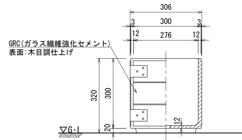
側・断面図
