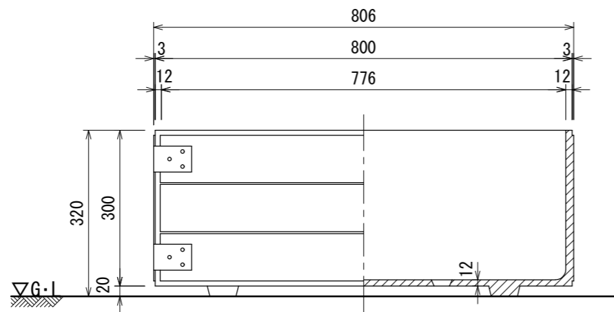
立・断面図
