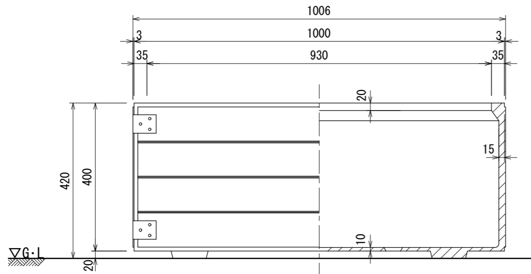
立・断面図
