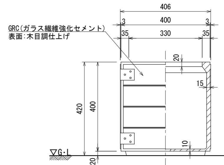
側・断面図
