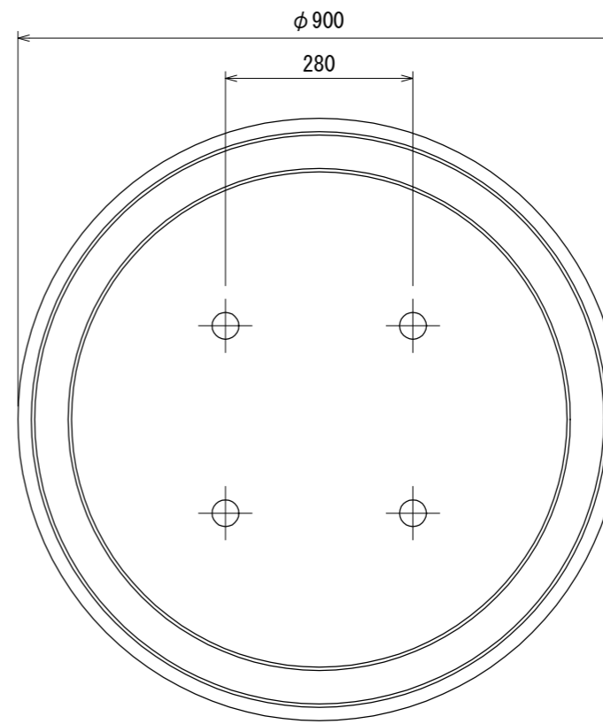
底面図
