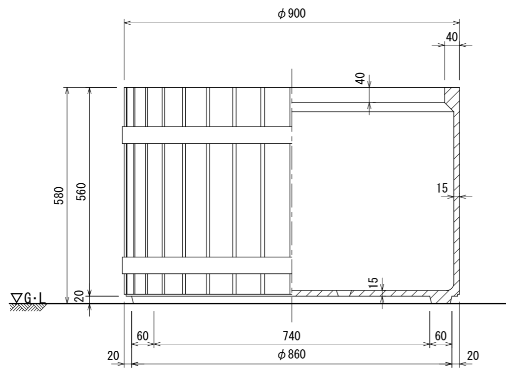
立・断面図
