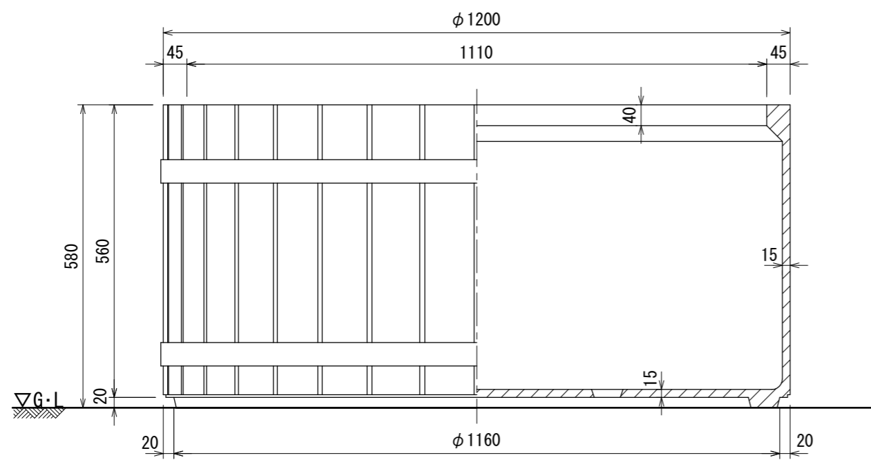
立・断面図
