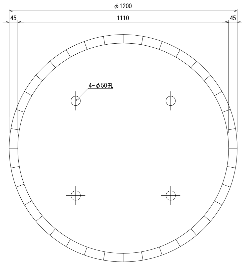
平面図
