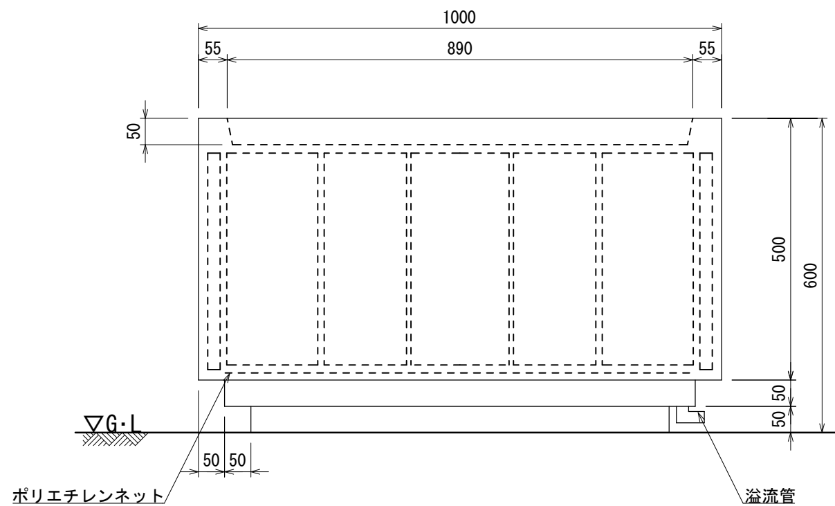
立面図
