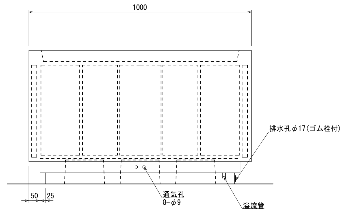
側面図
